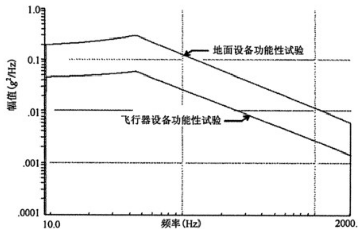
图 2 与图 1 等效的随机试验的输入 ASD
