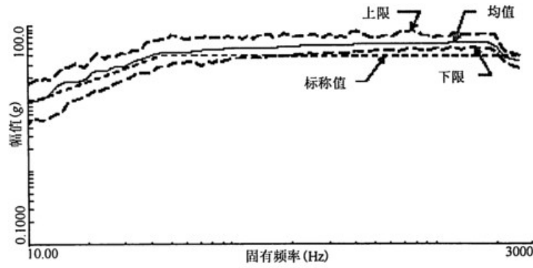
图 D.3 地面设备功能性试验的冲击响应谱比较
