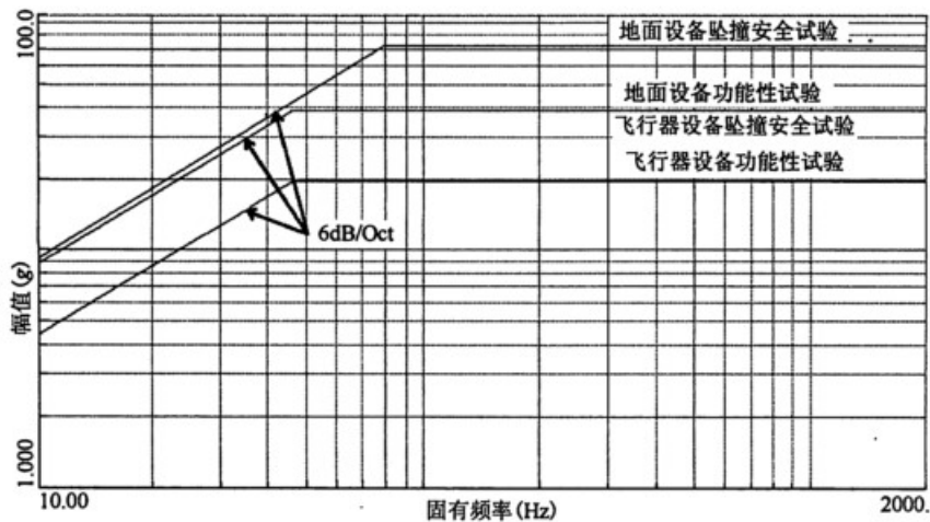
图 1 没有测量数据时使用的冲击响应谱
