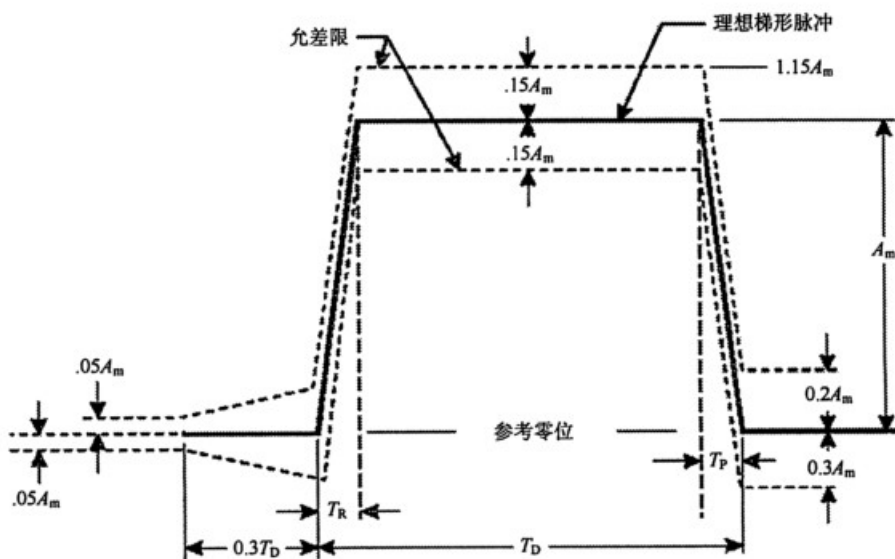
图 4 对称梯形脉冲波形参数和允差
